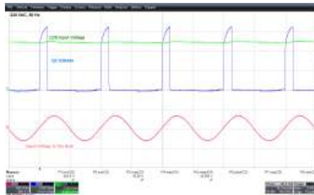
Figure 39 – 230 VAC, BLE Load.
