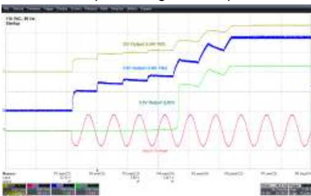
Figure 30 – 115 VAC, BLE Load.
